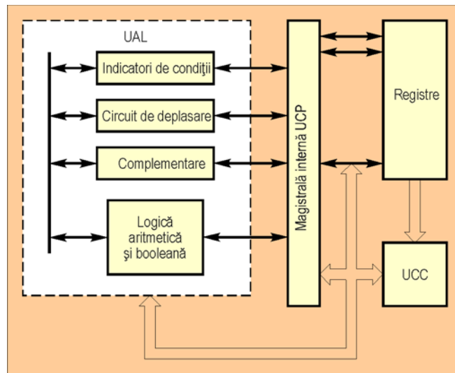
Structura mai detaliată a UCP
