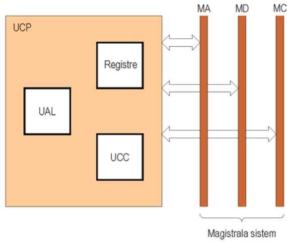
Structura generală a UCP împreună cu magistrala sistem
