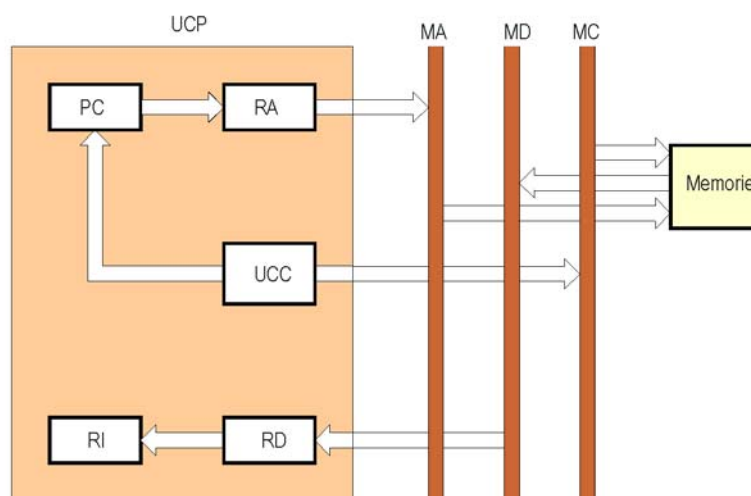
Transferuri de date în subciclu de extragere
