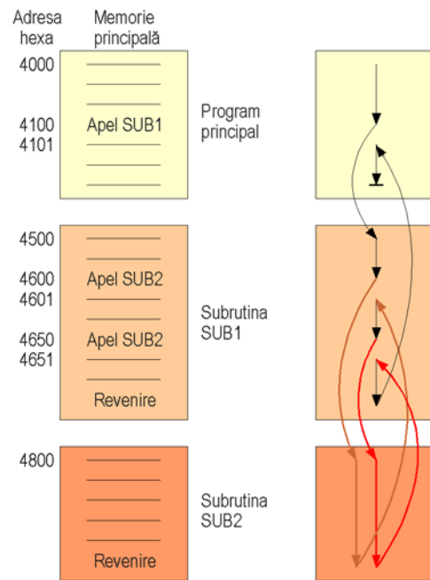
Execuția subrutinelor dintr-un program
