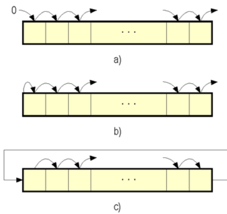
Ilustrarea operațiilor de deplasare și rotire la dreapta: (a) deplasare logică la dreapta; (b) deplasare aritmetică la dreapta; (c) rotire la dreapta
