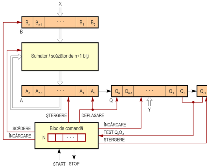
Schema bloc a unui dispozitiv de înmulțire prin metoda Booth
