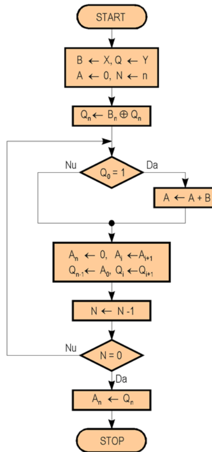
Organigrama operației de înmulțire prin metoda directă
