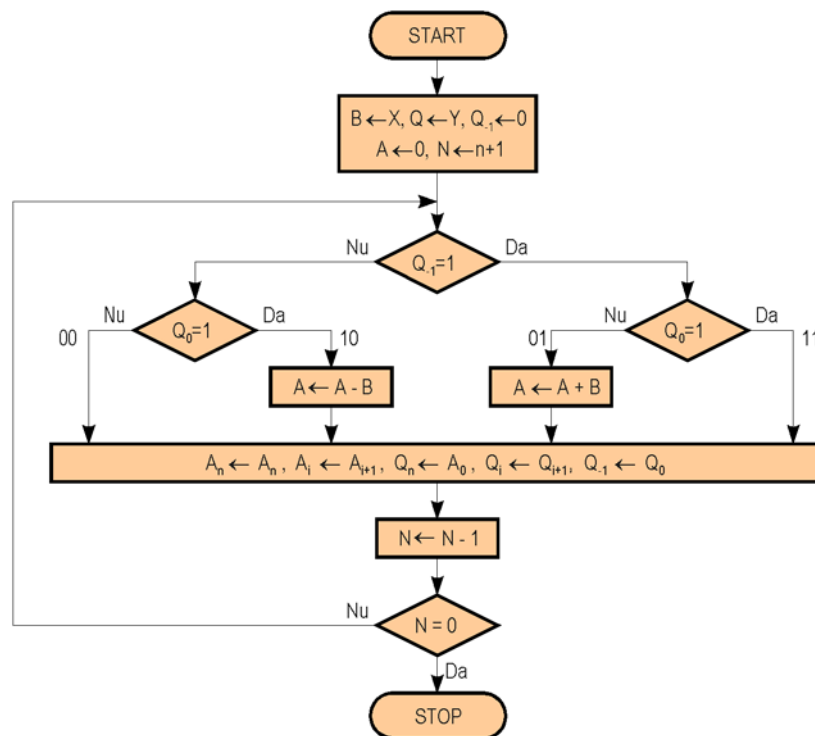
Organigrama operației de înmulțire prin metoda Booth
