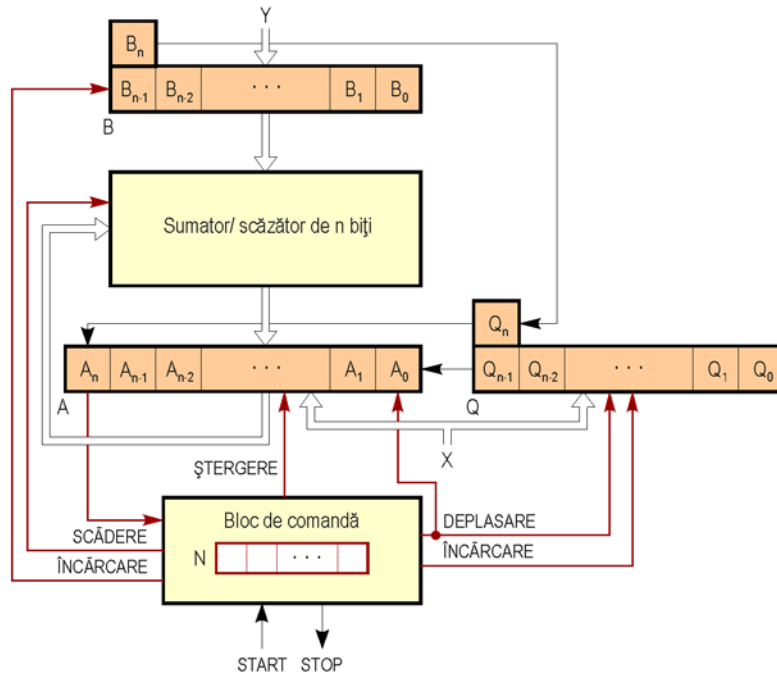
Schema bloc a unui dispozitiv de împărțire prin metoda refacerii restului parțial
