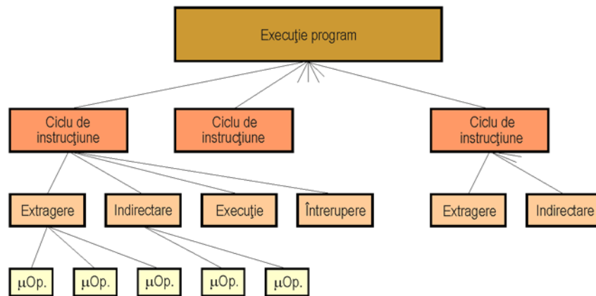
Elementele componente ale execuției unui program
