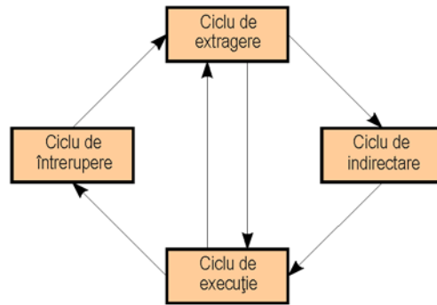
Ciclul de instrucțiune
