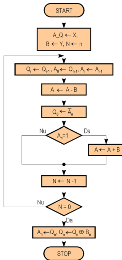
Organigrama operației de împărțire prin metoda refacerii restului parțial
