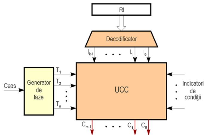
Structura generală a unei unități de comandă și control care utilizează un decodificator
