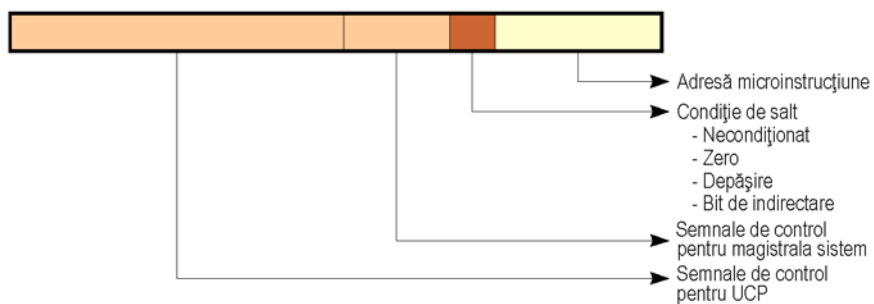
Format tipic de microinstrucțiune orizontală
