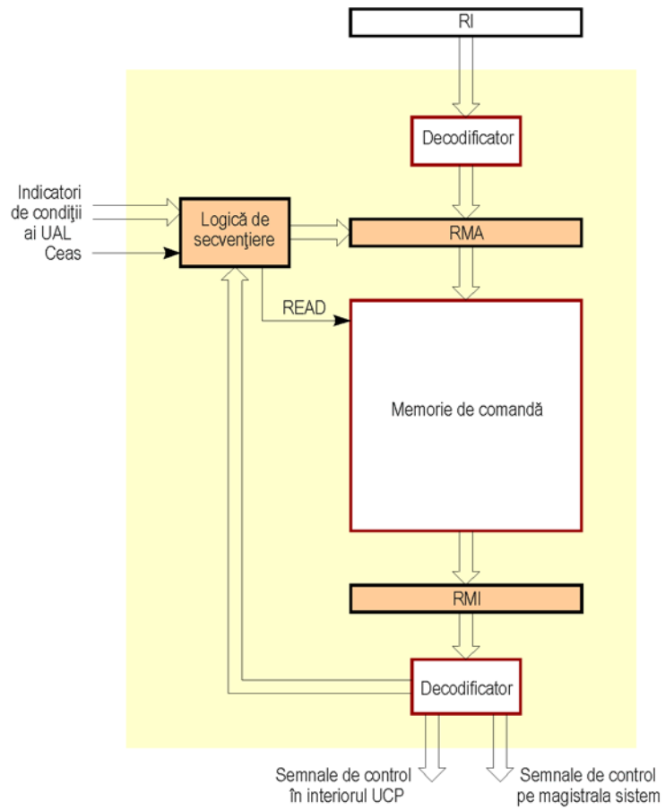
Structura mai detaliată a unei unități de comandă microprogramate
