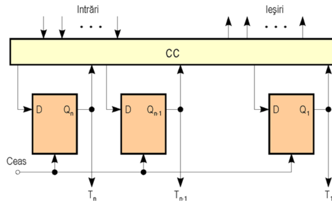
Structura generală a unei unități de comandă și control care utilizează un bistabil pe stare
