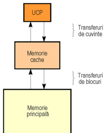
Principul memoriei cache
