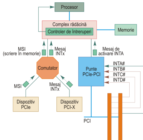
Figura 2.7. metode de semnalare a întreruperilor într-un sistem PCIe.
