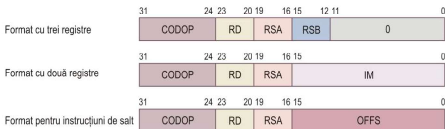
Figura 8.2. Formatele de instrucțiuni ale procesorului RISC.
