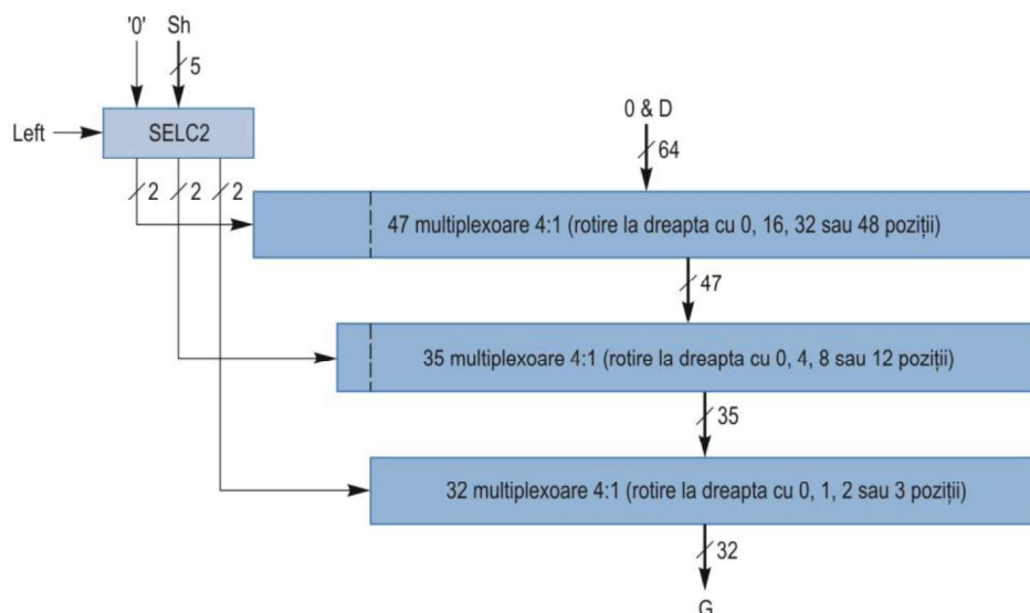
Figura 8.5. Schema bloc a circuitului combinational de deplasare de 32 de biți.
