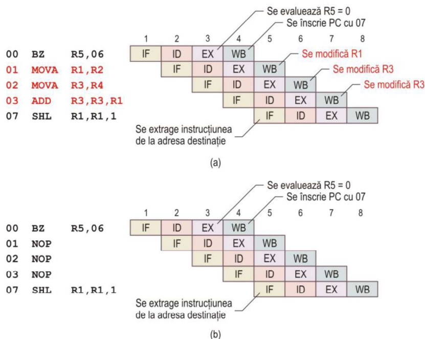
Figura 8.6. Exemplu de hazard de control: (a) ilustrarea problemei hazardului de control; (b) eliminarea hazardului de control prin inserarea unor instrucțiuni NOP.
