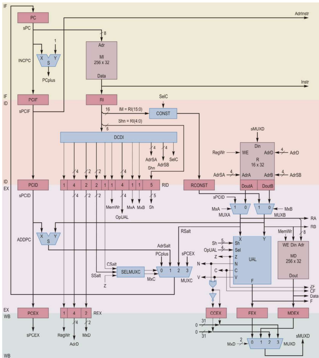
Figura 8.3. Schema bloc detaliată a procesorului RISC.
