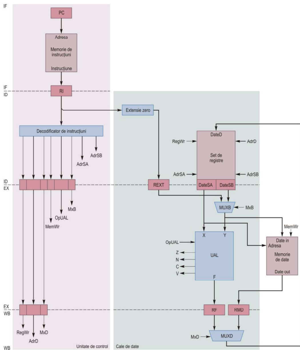
Figura 8.1. Schema bloc simplificată a unității de control și a căii de date pentru procesorul RISC.
