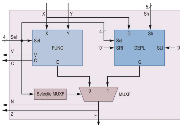
Figura 8.4. Schema bloc a unității aritmetice și logice.
