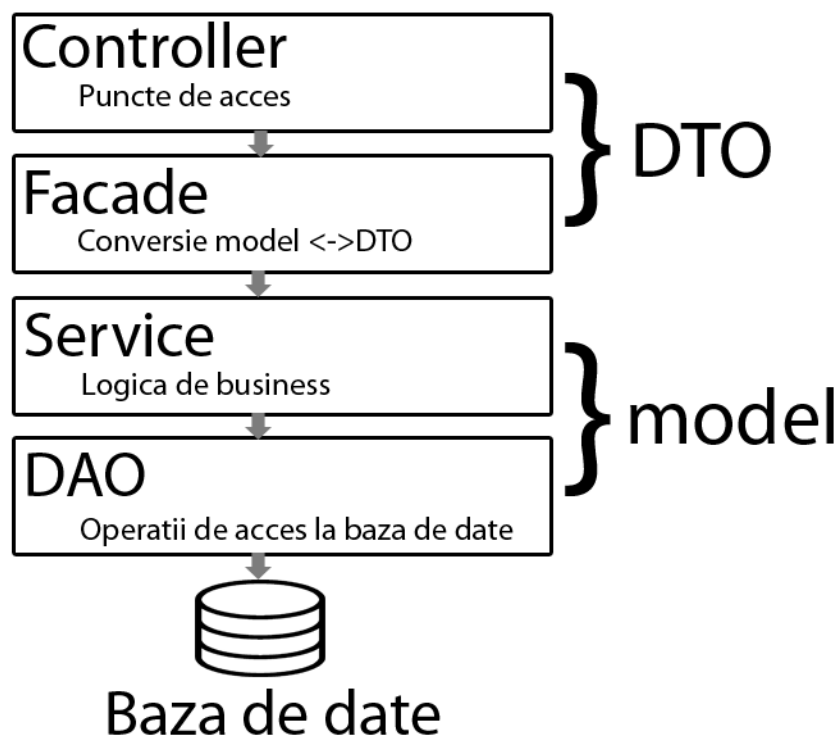
Figura 5.3 Arhitectura backend
