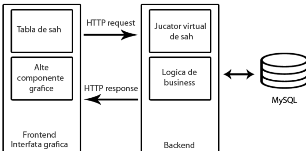
Figura 5.1 Arhitectura sistemului
