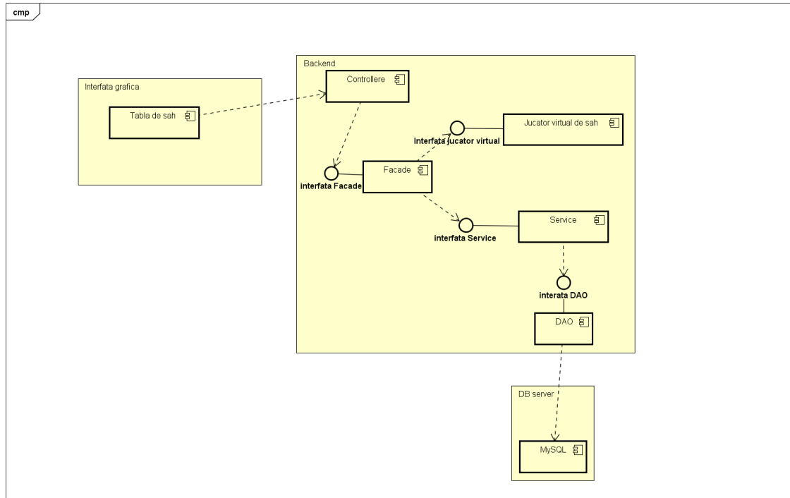
Figura 5.2 Diagrama de componente a sistemului
