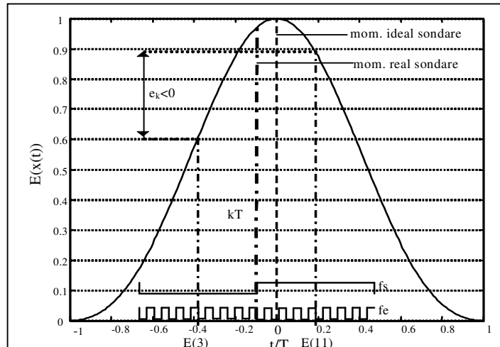
Figura 9.b Relația între E(3) și E(11) pentru tactul local de simbol defazat înaintea semnalelor demodate
