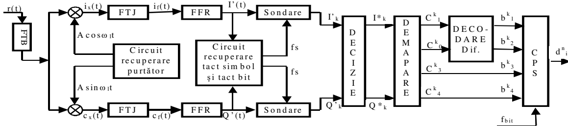
Figura 3. Schema bloc a demodulatorului ASK+PSK realizat prin metoda MAQ; varianta cu filtre trece-jos
