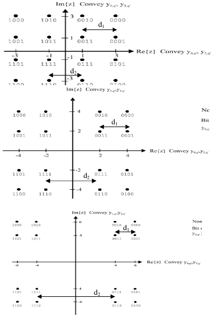
Figura 1. Constelațiile 16-QAM pentru f = 1, 2 sau 4 .
