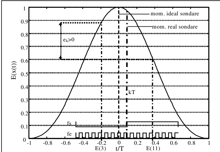
Figura 9.a Relația între E(3) și E(11) pentru tactul local de simbol defazat în urma semnalelor demodate
