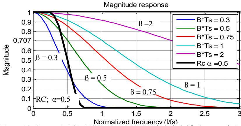
Figura 11. Caracteristicile G(f/f_s) pentru câteva valori ale lui \beta și caracteristica RC pentru \alpha=0.5
