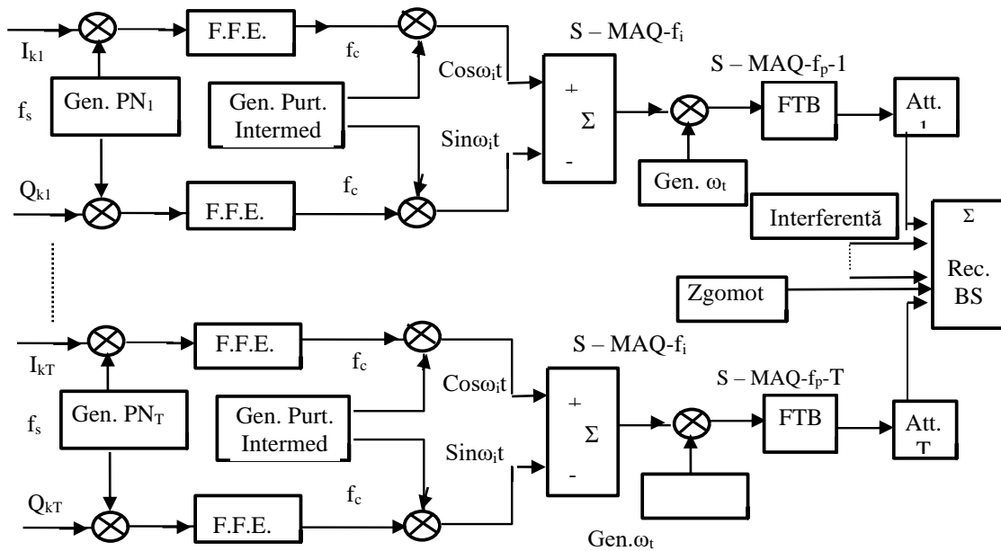
Figura 4. Suma semnalelor recepționate de stația de bază în UL - reprezentare schematică
