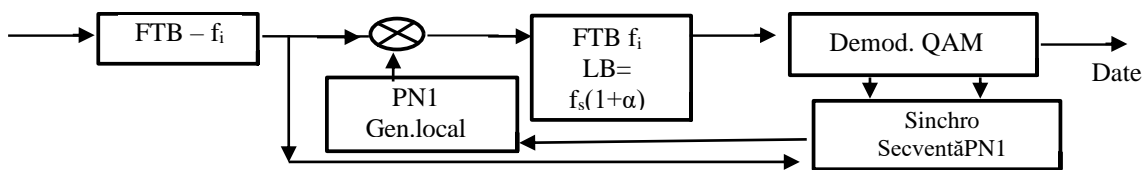
Schema bloc a receptorului DS-SS UT and BS
