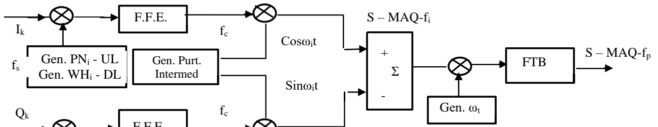
Fig.1. Schema bloc generică a modulatorului DS-SS -DL și UL
