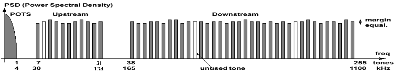
Fig. 14. Dispunerea spectrală a legăturii ADSL cu DMT
