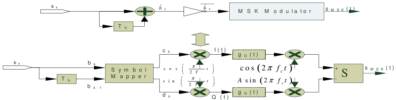
Figura 7. Principiul “precoded MSK” Schema bloc a modulatorului “precoded MSK”
