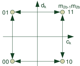
Figura 6. Reprezentarea spațiului semnalului MSK
