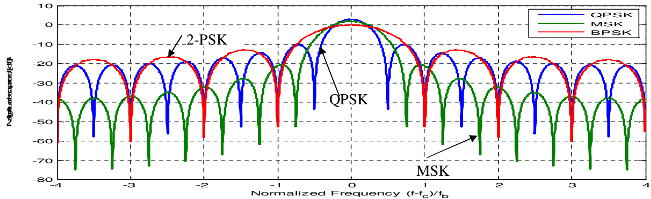
Figura 3.b. PSD ale semnalelor MSK, 2-PSK, QPSK
