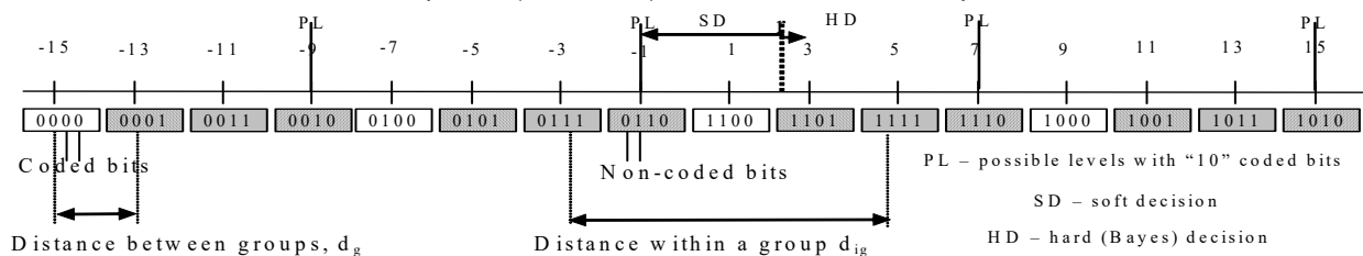
Figura 29. Maparea biților pe o axă a constelației și decizia soft a biților necodați
