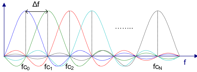
Figura 6. Suprapunerea spectrală a semnalelor OFDM.
