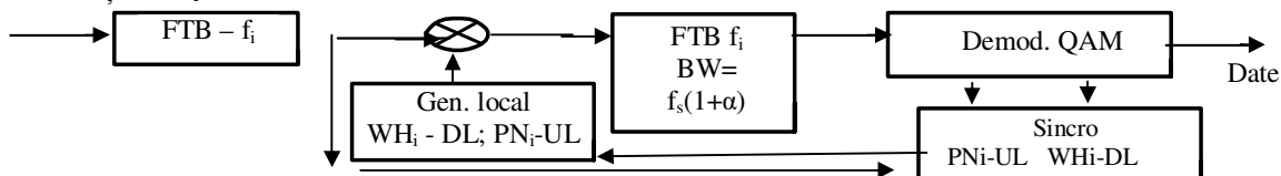
Figura 2. Schema bloc a demodulatorului DS-SS - UT și BS
