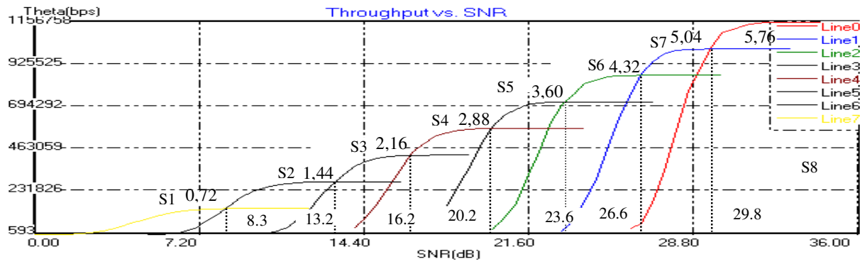
Eficiențele configurațiilor din setul NC, tabelul 1. Constanta K=0.72 , R_{cfr}=1 , BW_{ch}=200,826 kHz
