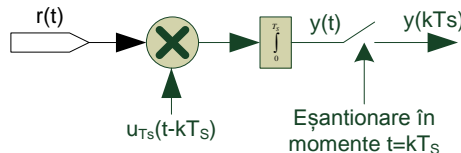
Figura 3. Demodulare PAM cu intercorelator
