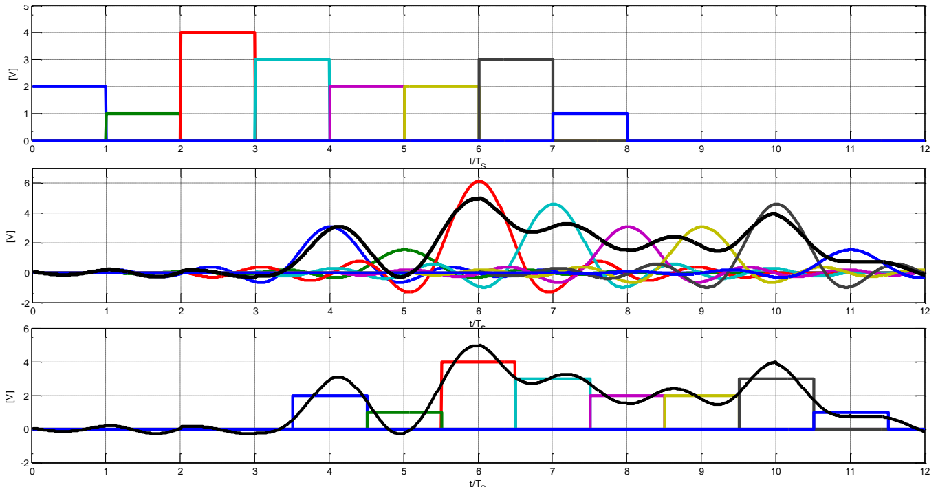
Figura 5 Filtrarea trece jos a impulsurilor. a). nivele de intrare. b). impulsurile individuale filtrate. c). Semnalul original și semnalul filtrat
