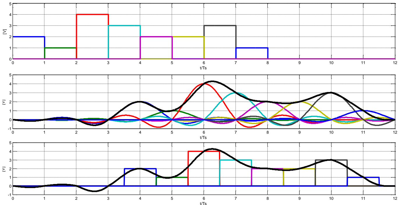
Figura 10 Filtrarea trece jos a impulsurilor cu un filtru Nyquist.
