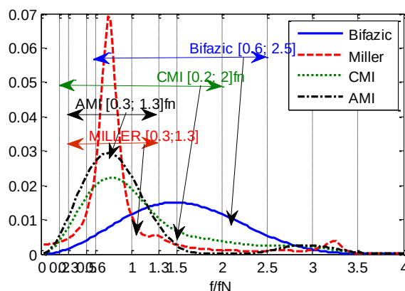
Figura 2. Densitatea spectrală de putere a codurilor bifazic-S, Miller, CMI și AMI
