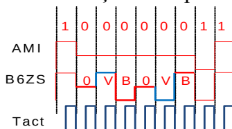
Figura 12. Exemplu de codare cu codul B6Zs
