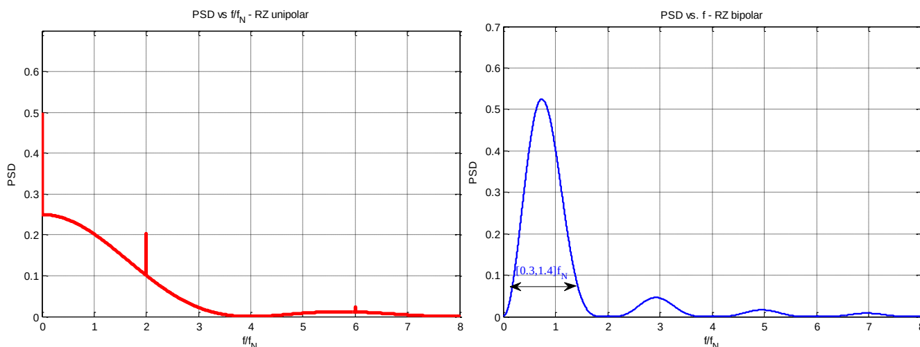
Figura 5. Densitatea spectrală de putere a codurilor RZ unipolar și RZ-bipolar
