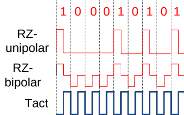
Figura 4. Exemplu de codare RZ
