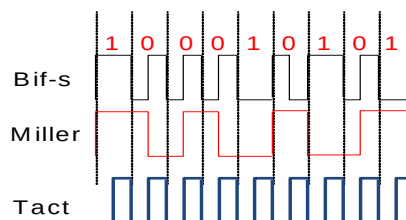
Figura 8. Exemplu de codare cu codul Miller
