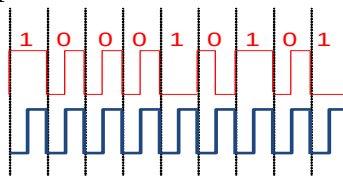
Figura 7. Exemplu de codare Bifazic-S
