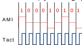
Figura 11. Exemplu de codare cu codul AMI
