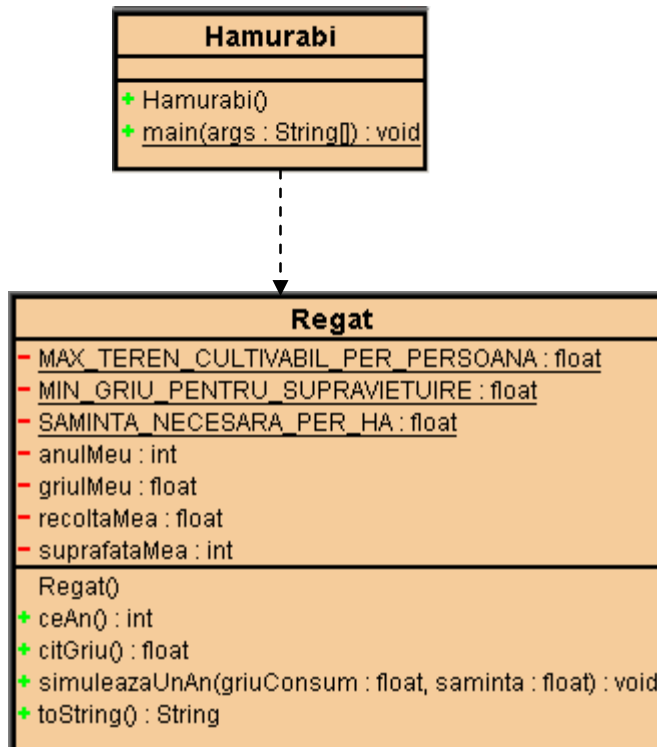
Diagrama de clase pentru proiectul de continuat Hammurabi
