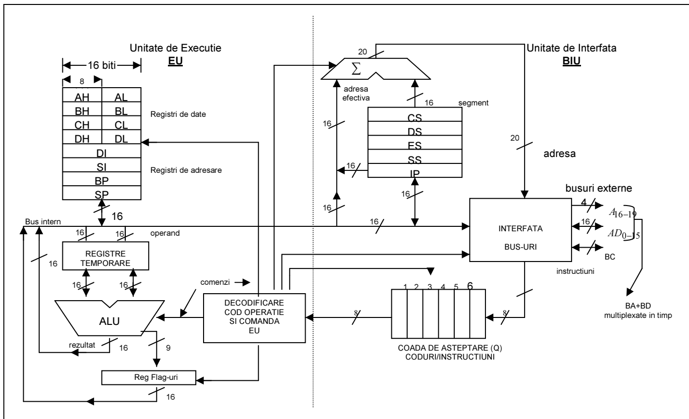
Fig. 4.3 Schema bloc internă simplificată a microprocesorului 8086
