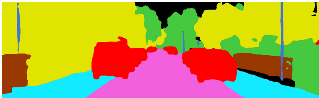
Segmentare semantică
